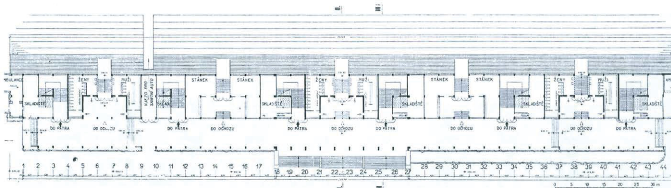
373 F. BALCÁREK—K. KOPP: Čprava jižního blešístě tribuny pro 10.000 osob, Půdorys 1:1000. — Устроителю южной трибуны для 10.000 зрителей. — Reconstruction of the South tribune for 10.000 spectators. — Adaptation de la partie sud de la tribune pour 10.000 spectateurs.
