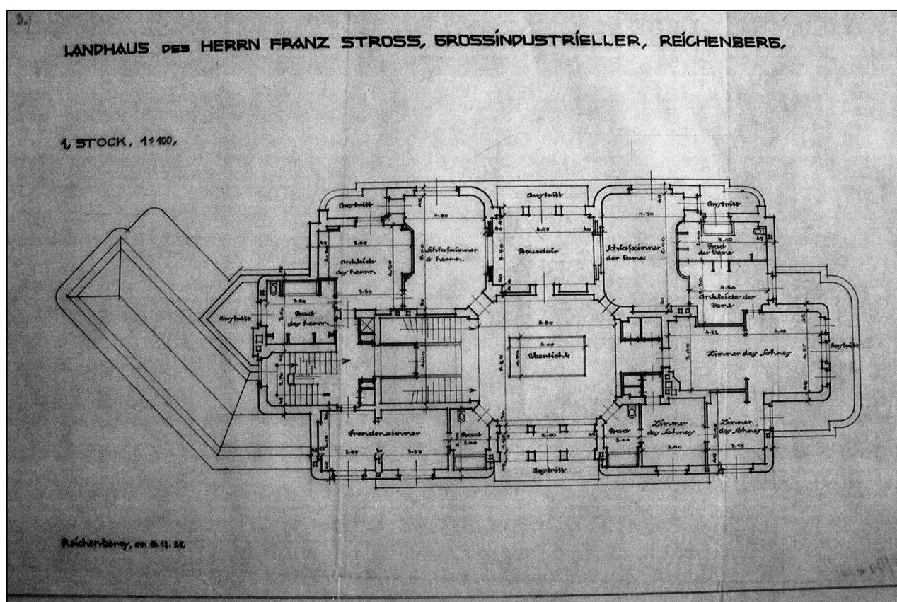
projekt domu č. p. 186, 16.12. 1925, architekt Thilo Schoder, půdorys 1. patra, Státní okresní archiv Liberec
