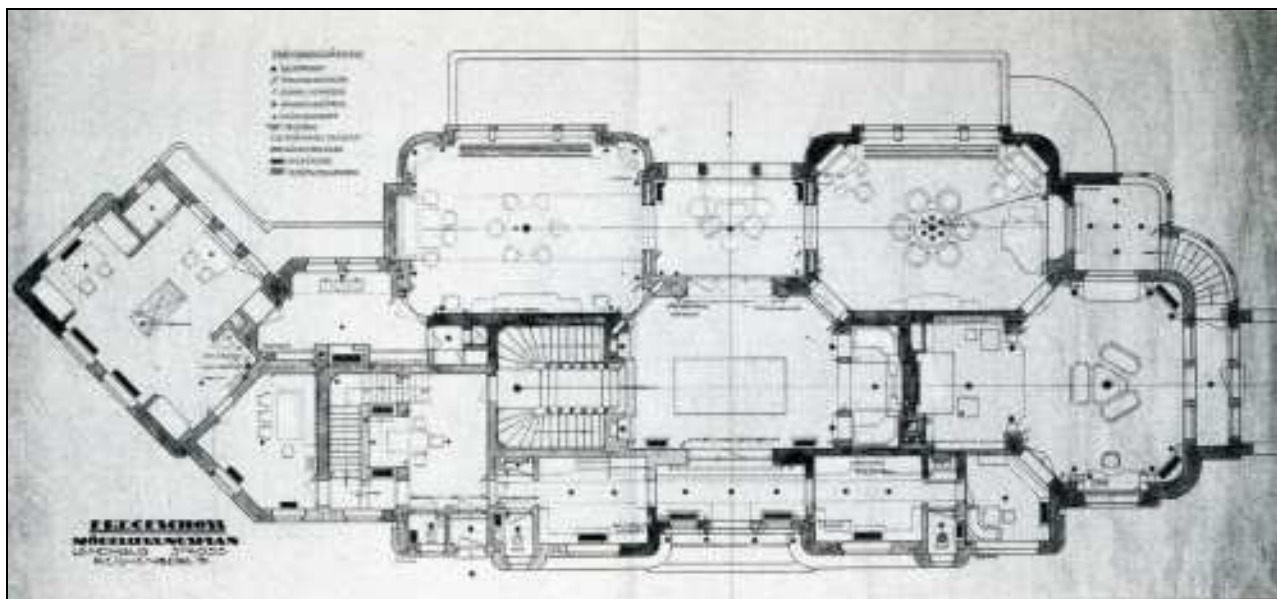
projekt domu č.p. 186, 1923, architekt Thilo Schoder, půdorys přízemí, Státní okresní archiv Liberec
