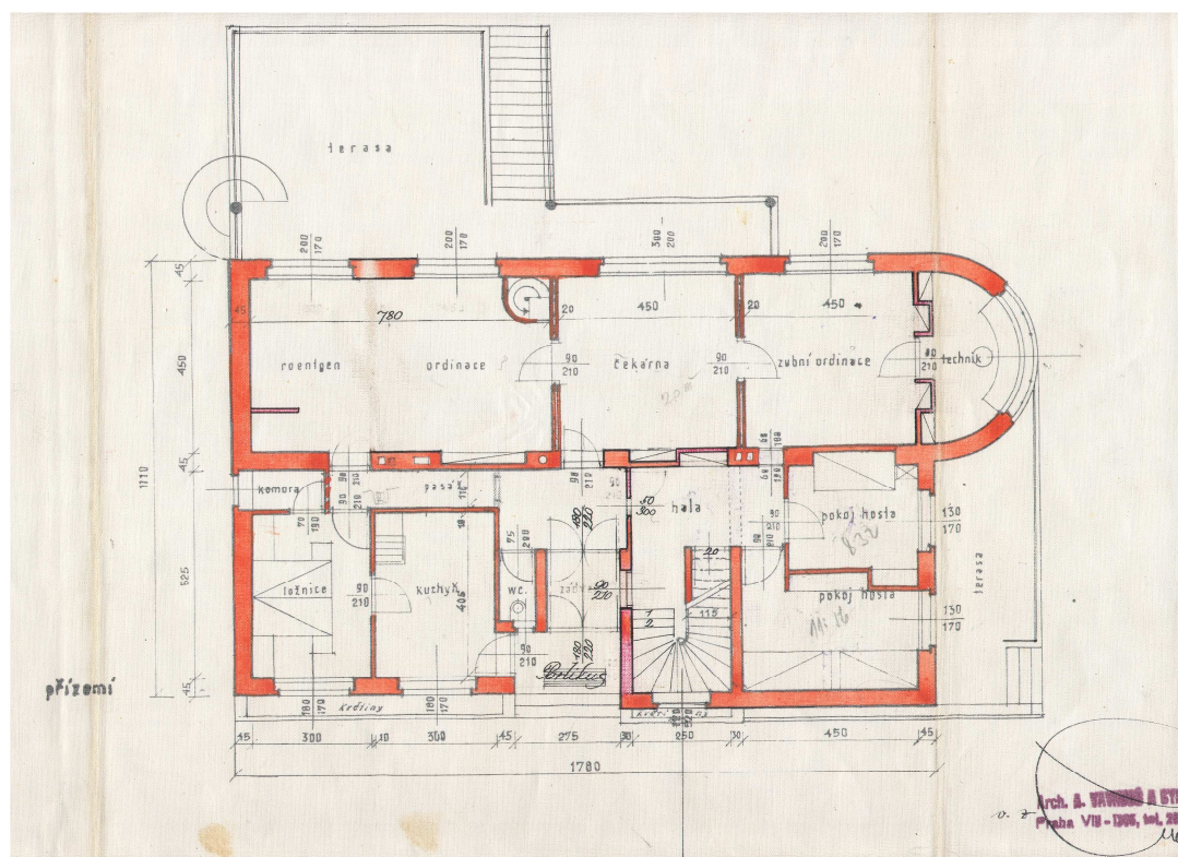
Řez a půdorys přízemí z nedatované plánové dokumentace signované Václavem Kolátorem a fi Alois Vavrouš a syn, stavební archiv MěÚ Jilemnice
