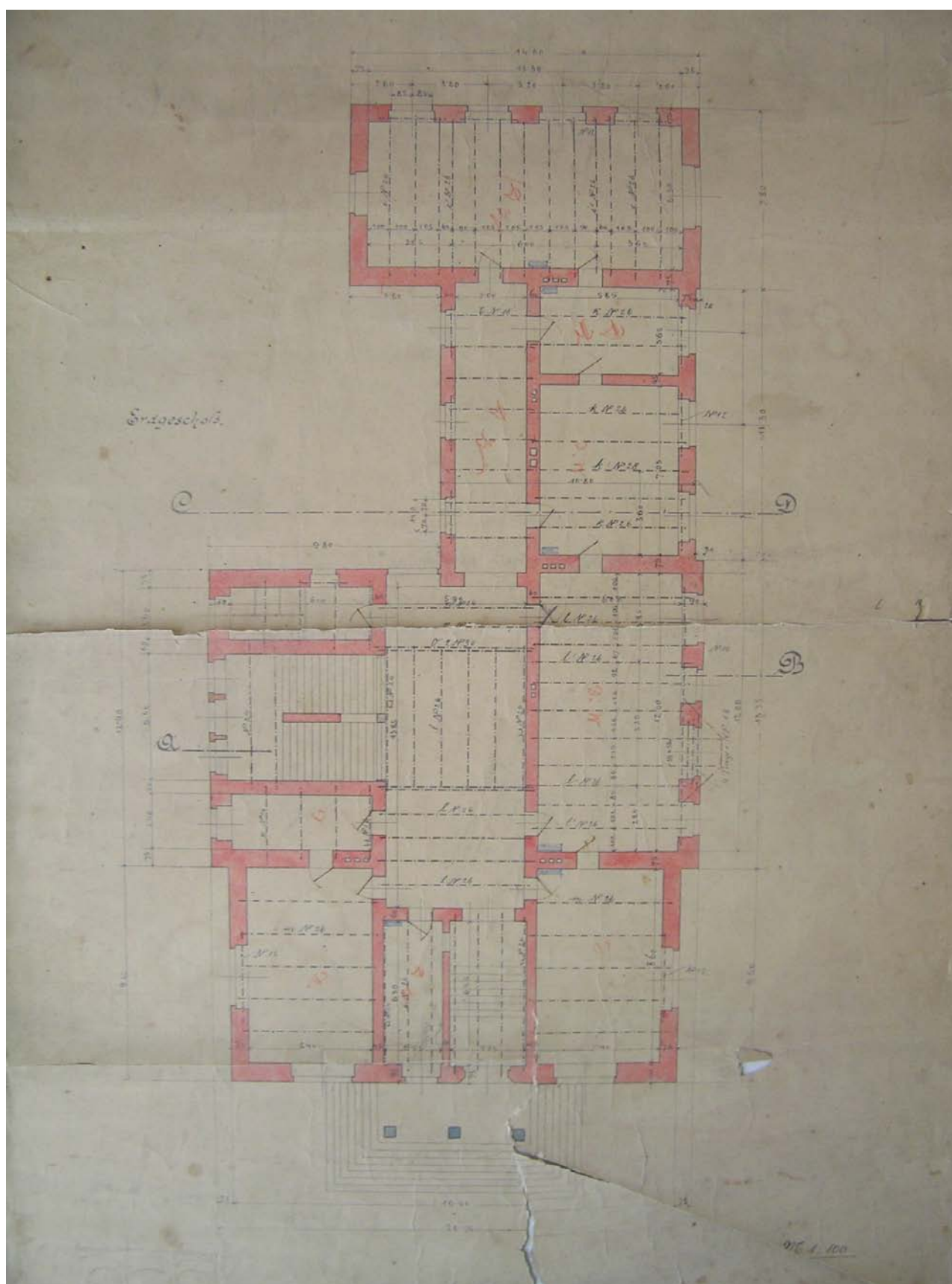
Obchodní a živnostenská komora v Liberci, půdorys přízemí.
