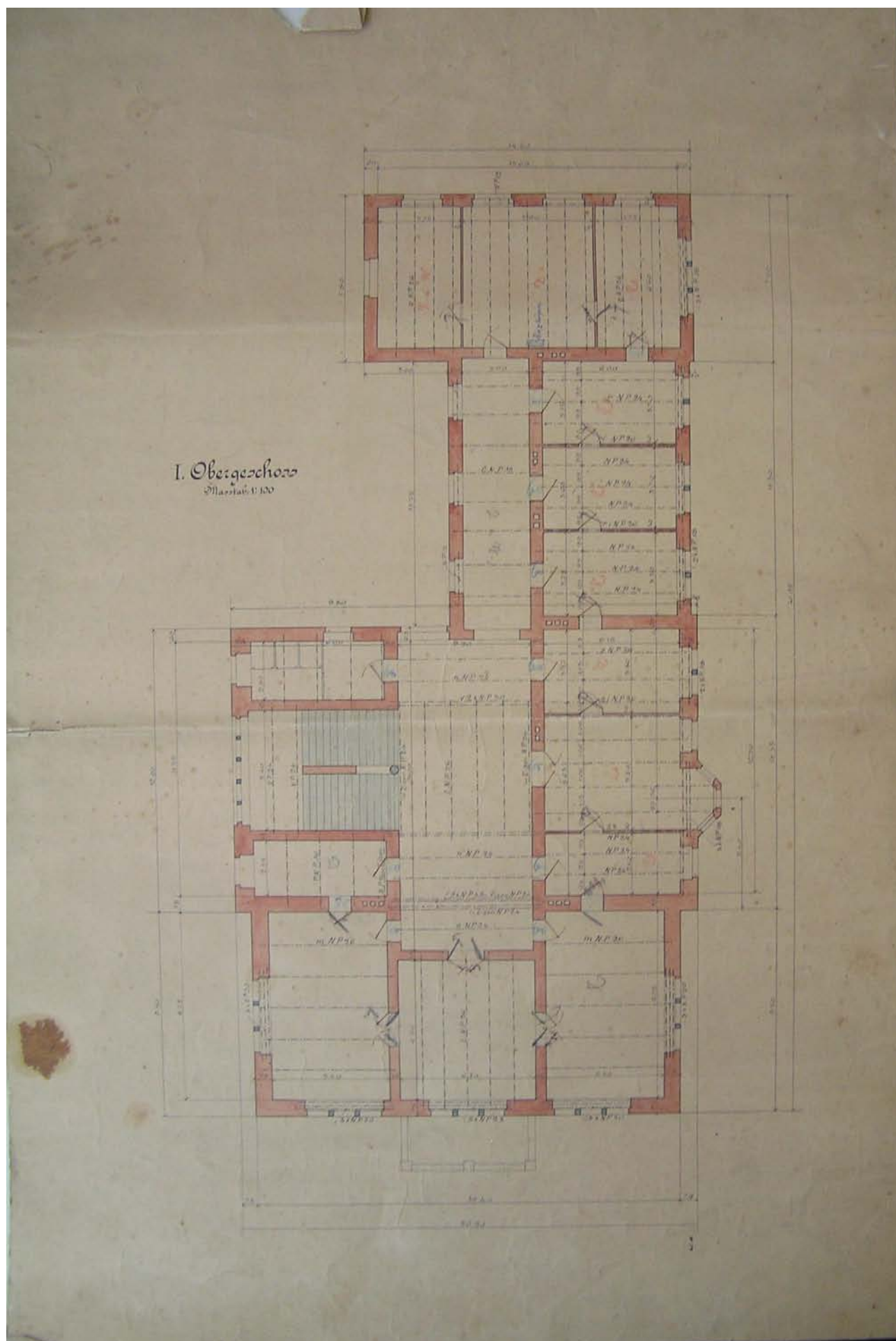
Obchodní a živnostenská komora v Liberci, půdorys prvního podlaží.
