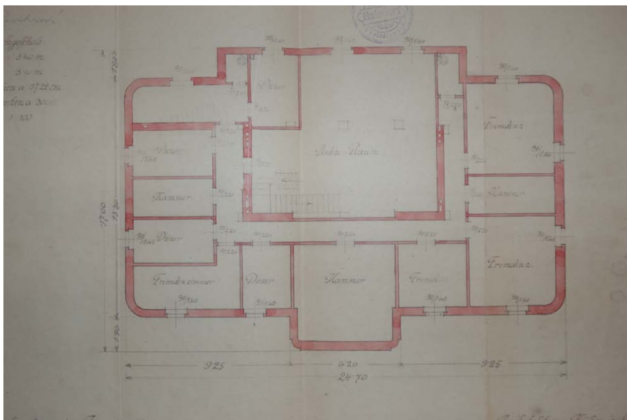
Půdorys podkroví vily čp. 435 na výřezu plánu z ledna 1907.
