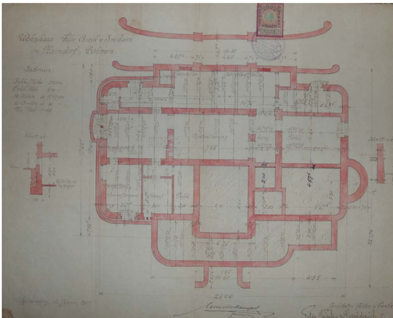
Půdorys suterénu vily čp. 435 na výřezu plánu z ledna 1907.
