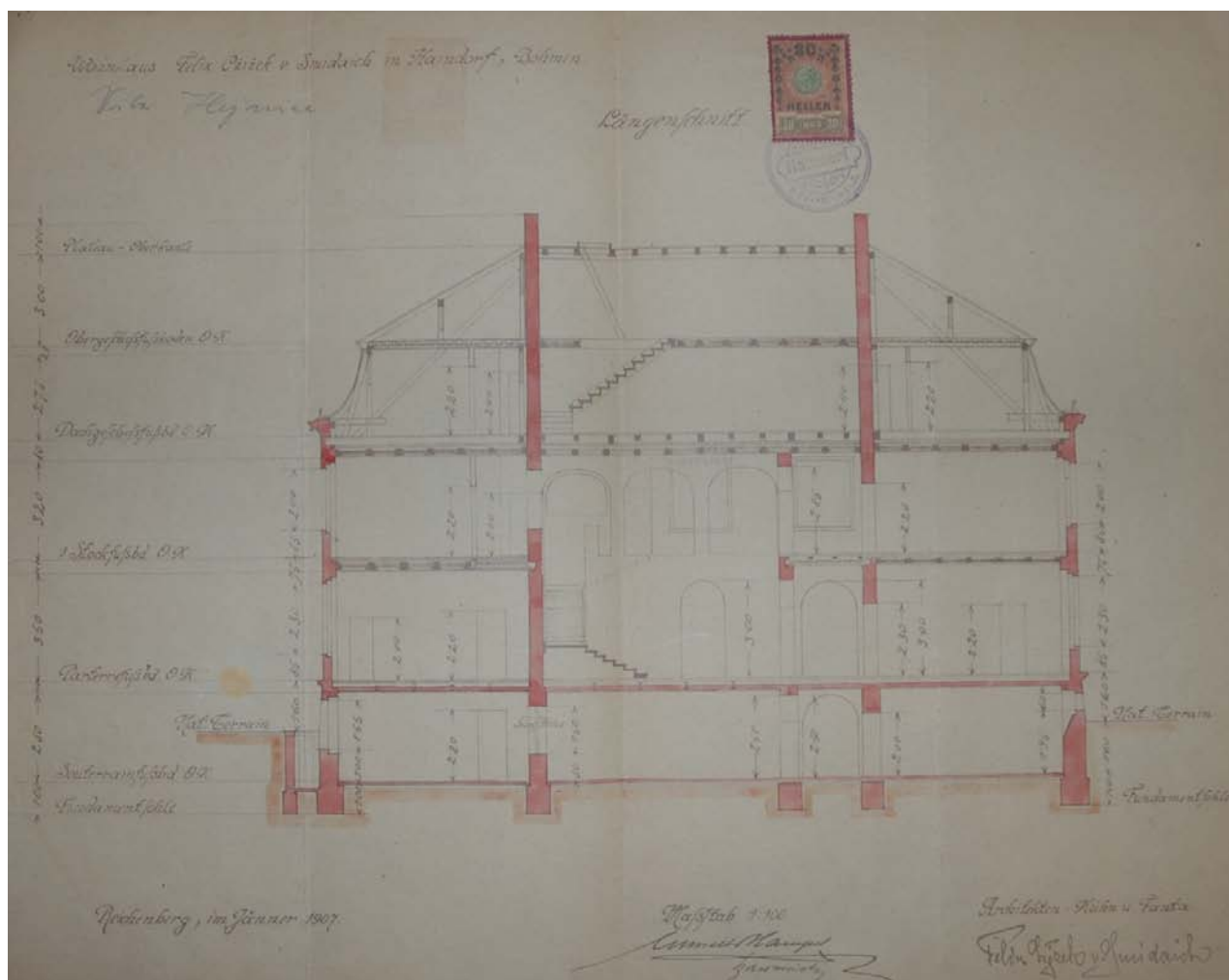
Řez vilou čp. 435 na výřezu plánu z ledna 1907.
