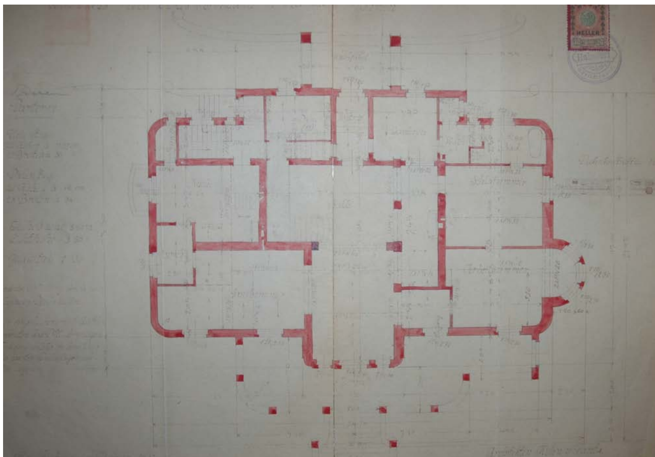
Půdorys přízemí vily čp. 435 na výřezu plánu z ledna 1907.
