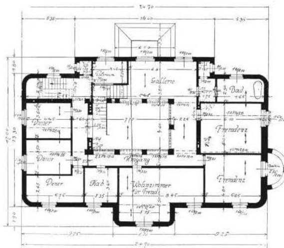
HERRENHAUS FELIX CZIŽEK VON SMIDAICH IN HAINDORF. HALLE UND I. STOCK- GRUNDRISS.
