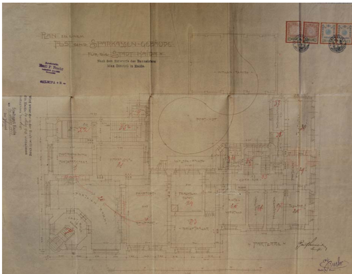
projekt domu č.p. 55 z roku 1903 od Emila Ruehra, půdorys přízemí, archiv stavebního úřadu MěÚ Nový Bor
