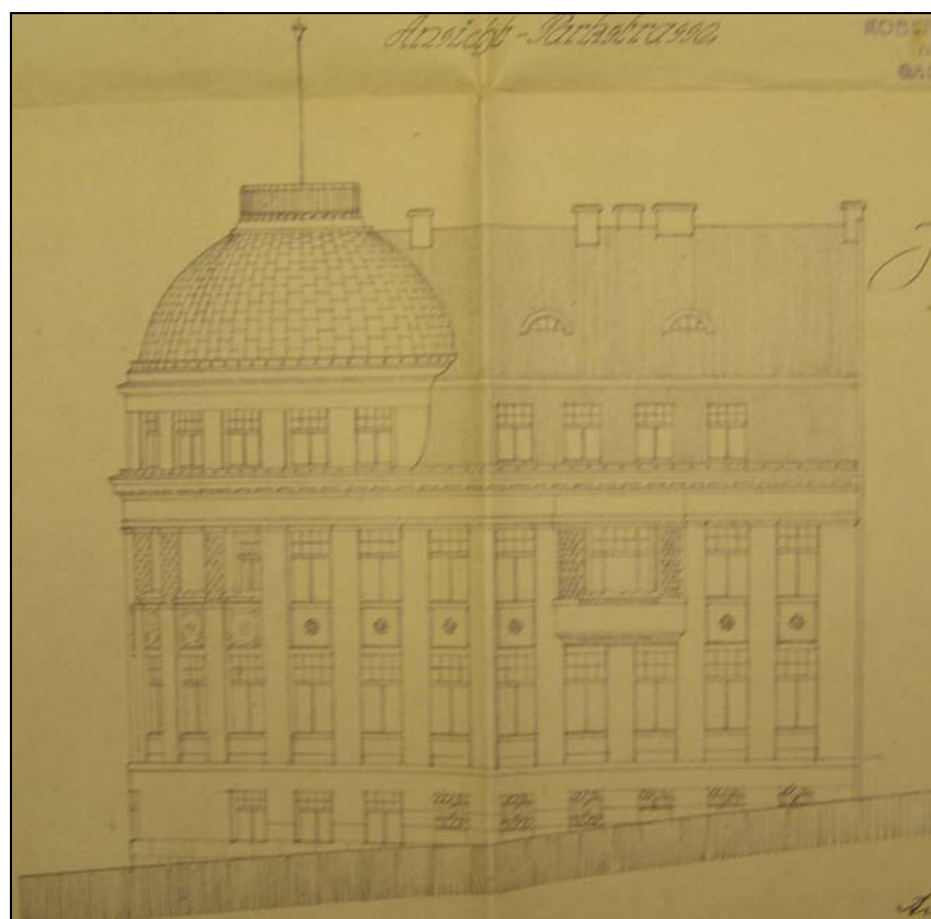
Projekt domu č.p. 145, R. Hemmrich 1924, západní fasáda, archiv SÚ Jbc
