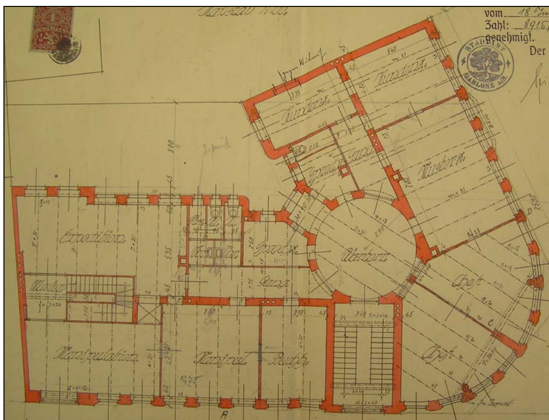
Projekt domu č.p. 145, R. Hemmrich 1924, 1. NP, archiv SÚ Jbc
