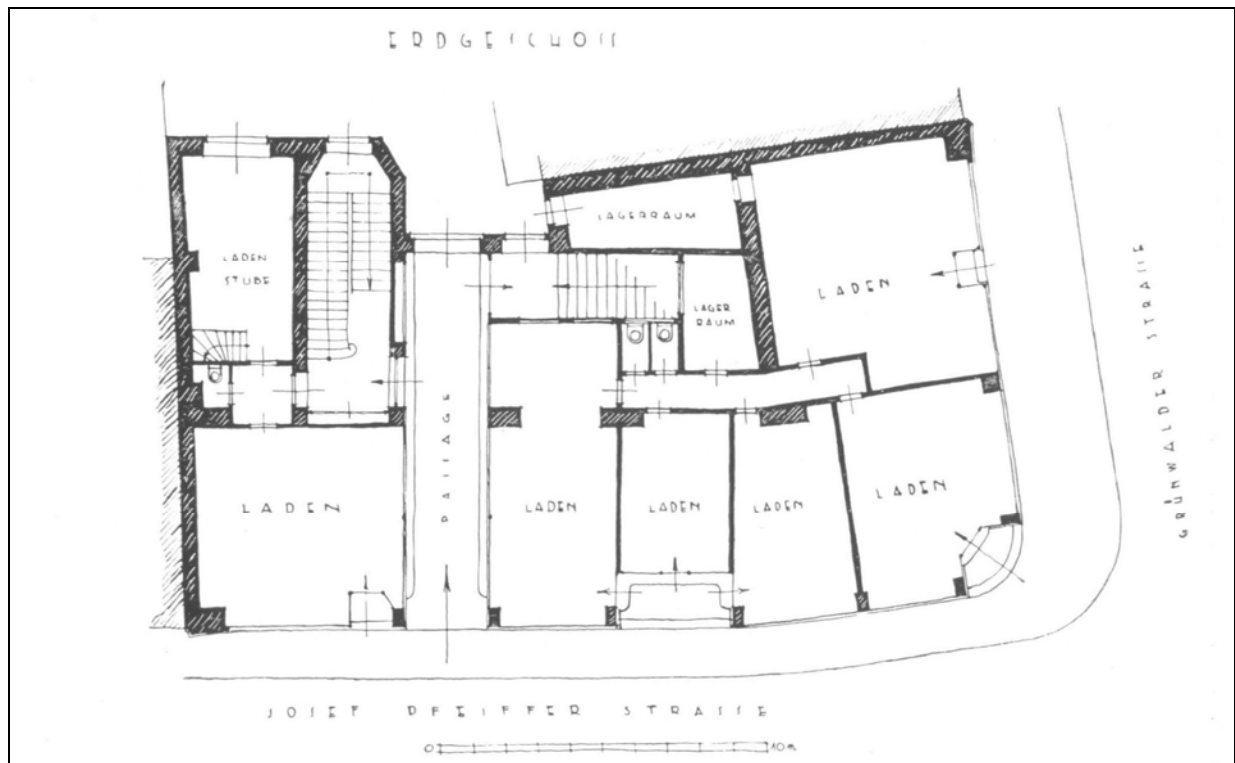
Wohn und Geschäftshaus E. K. in Gablonz a.N. (č.p. 91) - náčrtes 1. PP z publikace Ingenieur Architekt Rudolf Günter
