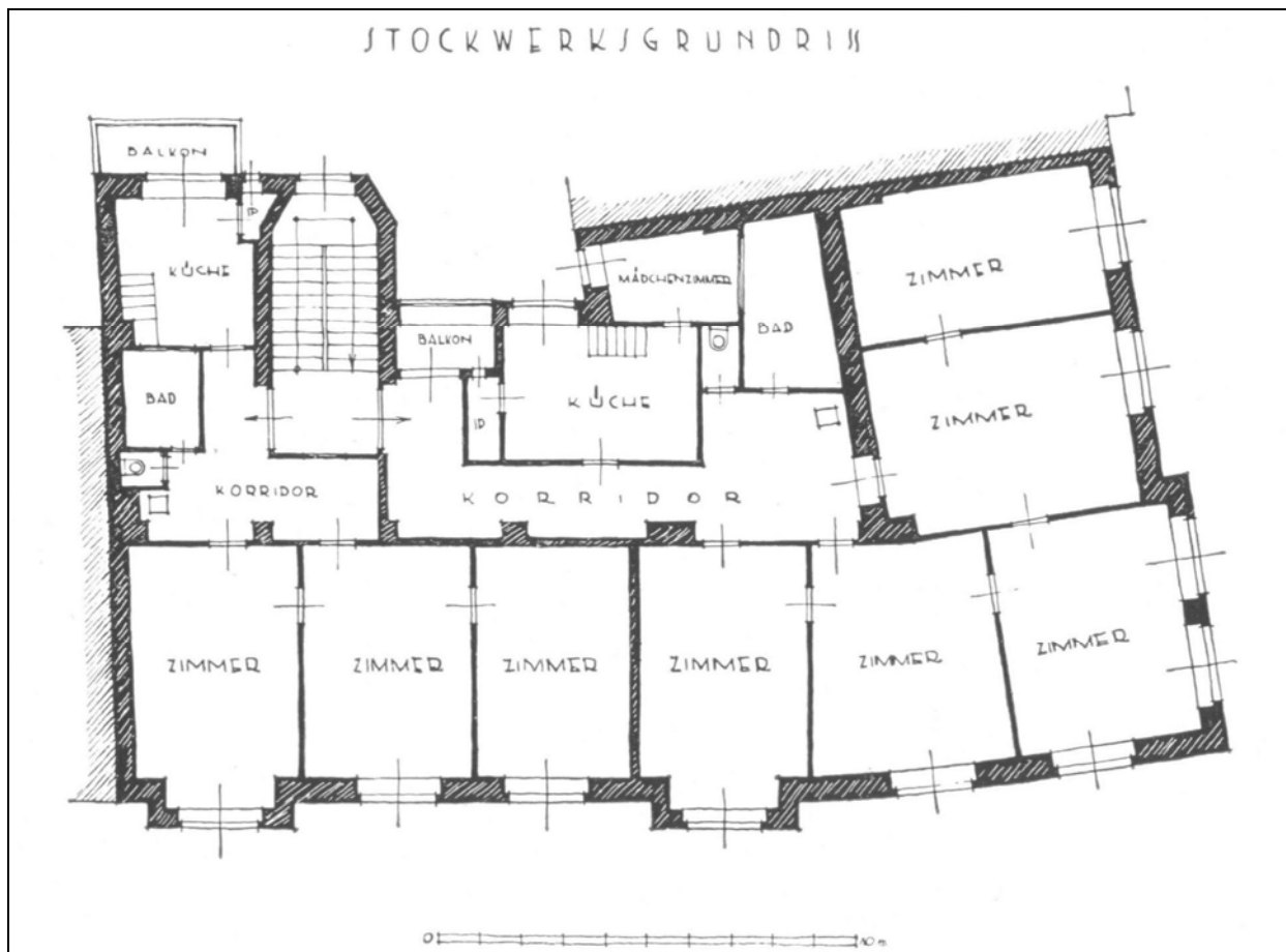
Wohn und Geschäftshaus E. K. in Gablonz a.N. (č.p. 91) - náčrtes patra z publikace Ingenieur Architekt Rudolf Günter
