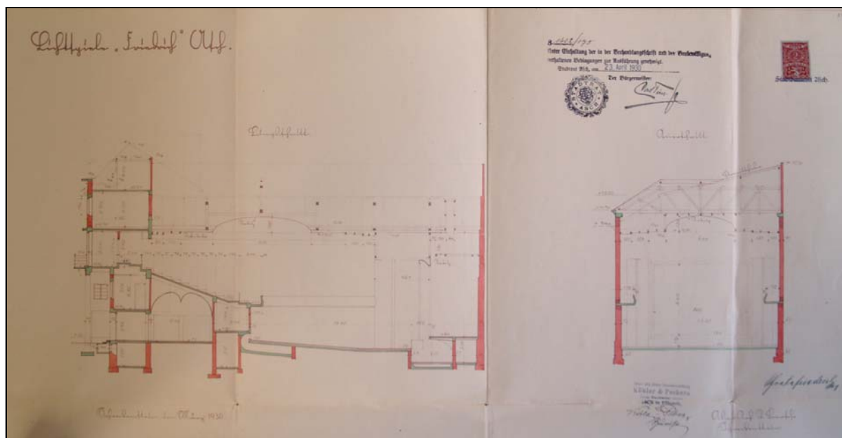
Aš, Masarykovo náměstí č.p. 1995, kino – plán stavby kina Friedrich, řezy, R. Brosche, Ústí nad Labem – Střekov leden 1930. Stavební archiv Městského úřadu Aš.
