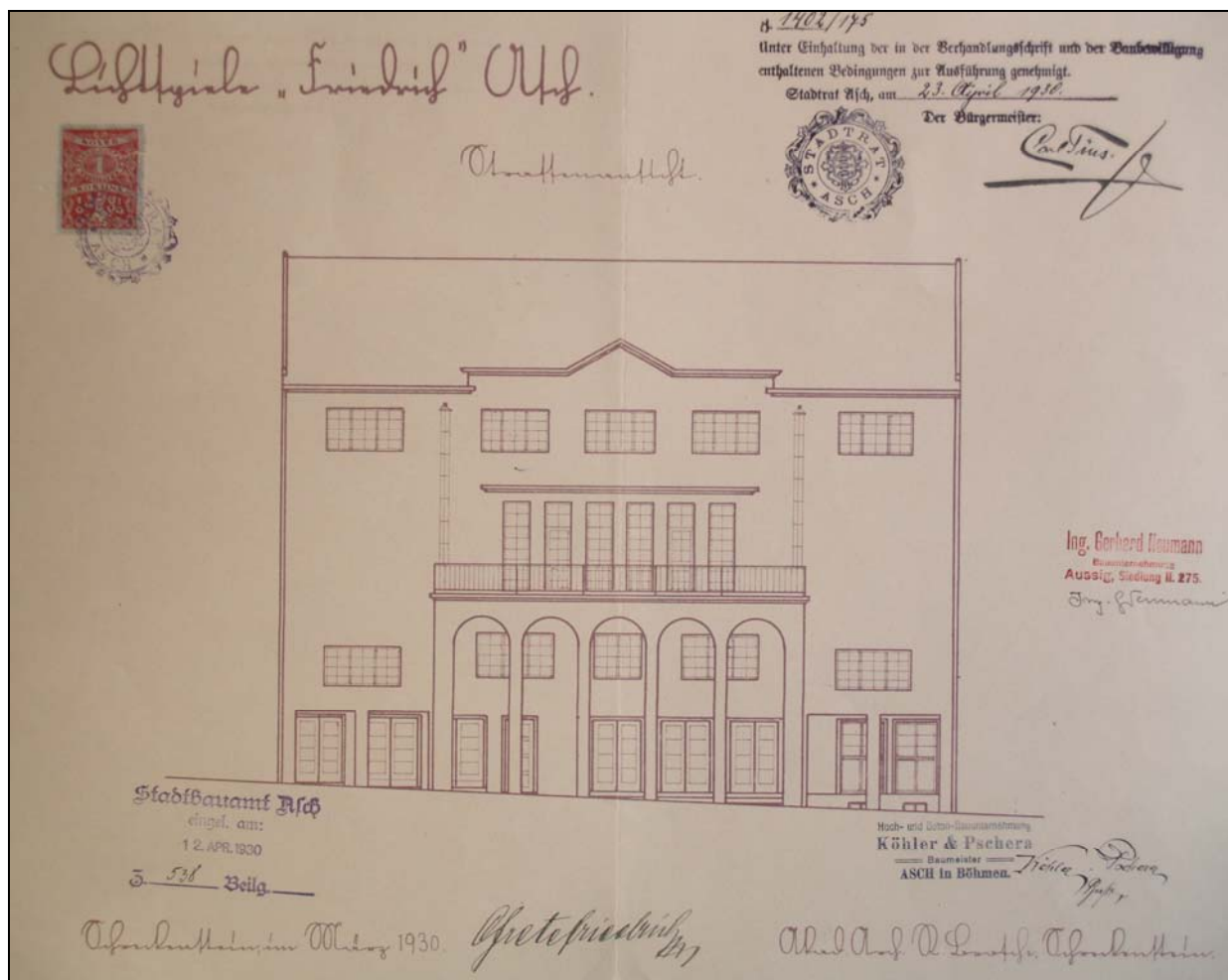
Aš, Masarykovo náměstí č.p. 1995, kino – plán stavby kina Fridrich, pohled, R. Brosche, Ústí nad Labem - Střekov, 1930. Stavební archiv Městského úřadu Aš.
