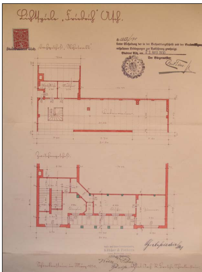
Aš, Masarykovo náměstí č.p. 1995, kino – plán stavby kina Friedrich, půdorys, R. Brosche, Ústí nad Labem – Střekov leden 1930. Stavební archiv Městského úřadu Aš.
