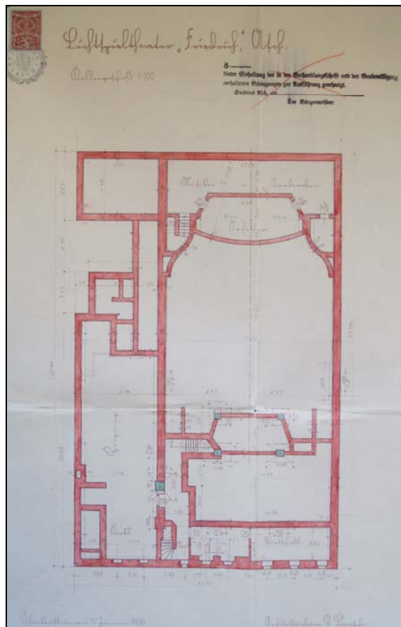
Aš, Masarykovo náměstí č.p. 1995, kino – plán stavby kina Fridrich, půdorys, R. Brosche, Ústí nad Labem - Střekov leden 1930. Stavební archiv Městského úřadu Aš.
