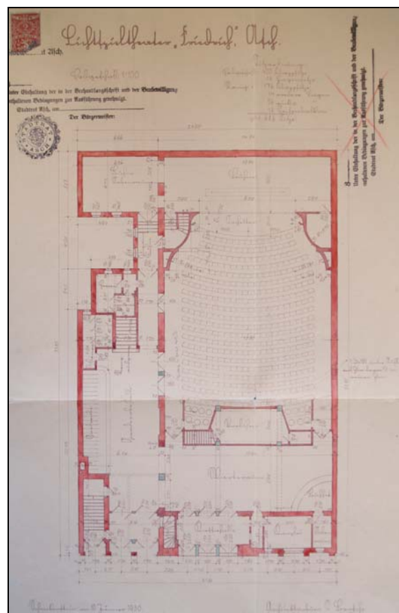
Aš, Masarykovo náměstí č.p. 1995, kino – plán stavby kina Friedrich, půdorys, R. Brosche, Ústí nad Labem – Střekov leden 1930. Stavební archiv Městského úřadu Aš.
