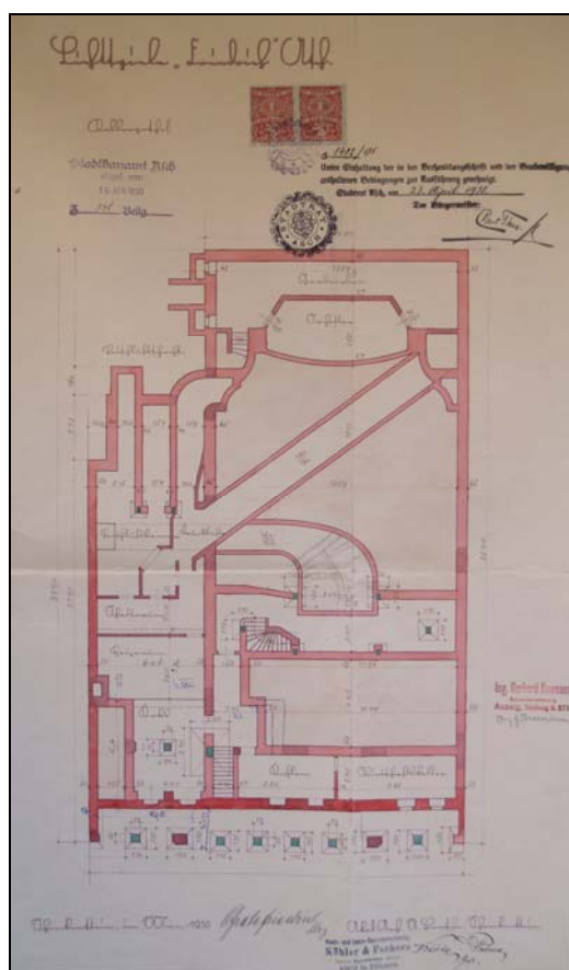
Aš, Masarykovo náměstí č.p. 1995, kino – plán stavby kina Fridrich, půdorys, R. Brosche, Ústí nad Labem- Střekov 1930. Stavební archiv Městského úřadu Aš.
