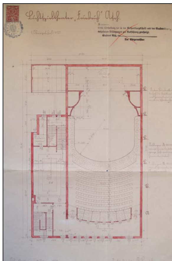
Aš, Masarykovo náměstí č.p. 1995, kino – plán stavby kina Friedrich, půdorys, R. Brosche, Ústí nad Labem – Střekov leden 1930. Stavební archiv Městského úřadu Aš.
