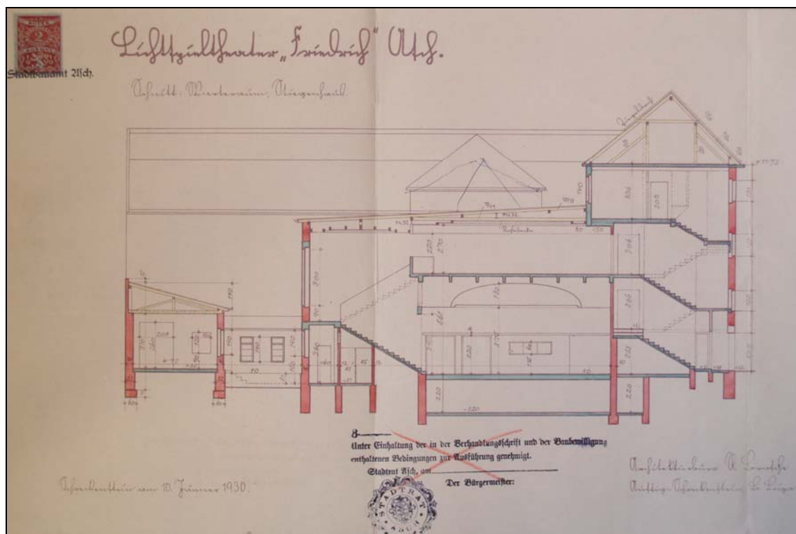
Aš, Masarykovo náměstí č.p. 1995, kino – plán stavby kina Fridrich, řez, R. Brosche, Ústí nad Labem - Střekov leden 1930. Stavební archiv Městského úřadu Aš.
